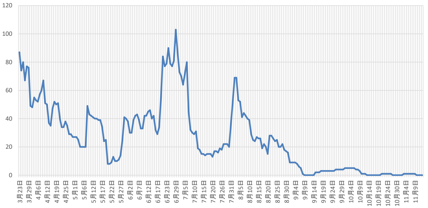
中央チカラン感染者推移(2021/11/14)
